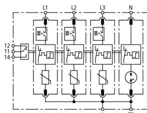
Kapcsolási rajz DG M TNS ACI 275 FM
