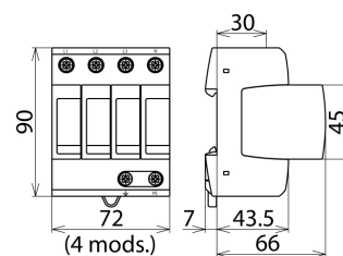
Beépítési méretek DG M TNS ACI 275 FM
